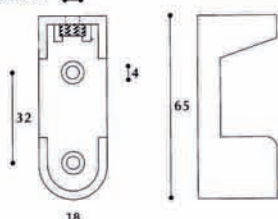
Art. 42180 Reggi tubo con dado 6M colori: bianco, marrone
