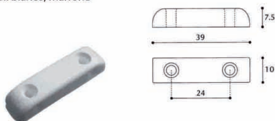
Art. 42004 Ferma porta forata colori: bianco, marrone
