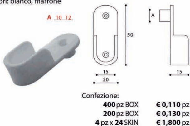
Art. 42080B Reggi tubo ovale codulo colori: bianco, marrone
