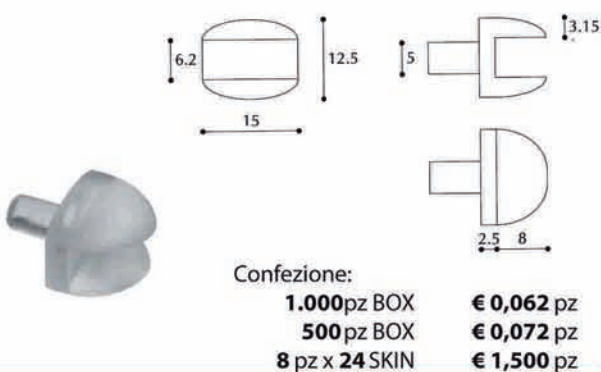
Art. 42258 Reggicristallo con O.R. colori: zincato
