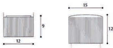
Art. 42009 Sostegno forato a vite ricoperto colori: bianco, marrone
