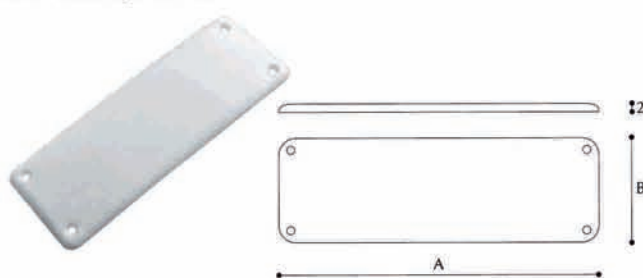
Art. 42007 Placca copri serrature colori: bianco, marrone
