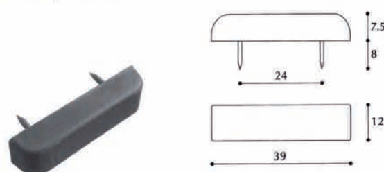
Art. 42005 Ferma porta pratic colori: bianco, marrone
