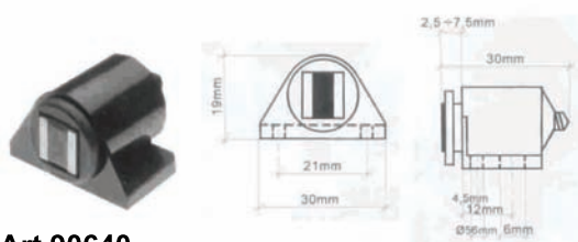
Art.90640 "magnetico regolabile" forza k 6
