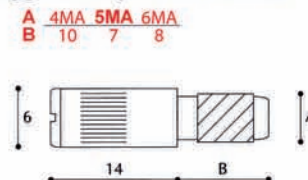
Art. 25503 Perno filettato per reggicristalli piani e a ventosa colori: zincato
