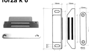
Art.90146 "magnetico" forza k 12
