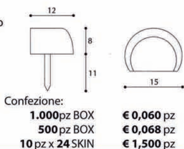
Art. 42094A Mensola con chiodo mobile ottonato colori: bianco, marrone
