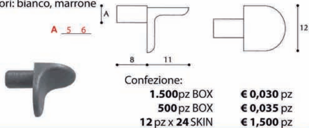
Art. 42029 Mensola cilindrica con anello colori: bianco, marrone
