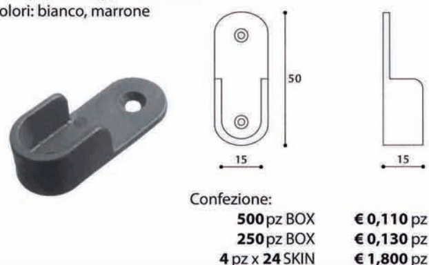
Art. 42080B Reggi tubo ovale codulo colori: bianco, marrone
