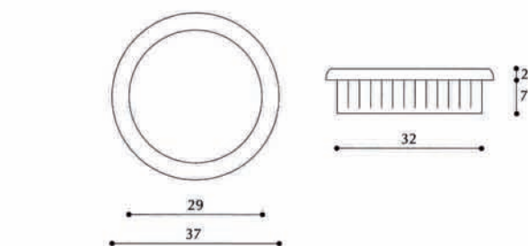
Art. 42020 Maniglia tonda colori: bianco, marrone, nero, grigio alluminio
