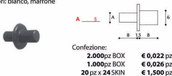
Art. 42028 Mensola con perno metallico colori: bianco, marrone, trasparente
