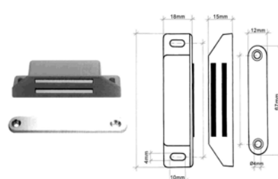
Art.91782 "magnetico" forza k 6
