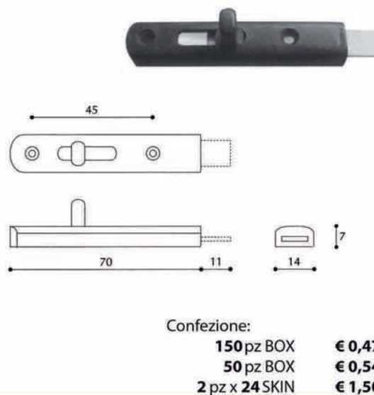
Art. 42122 Catenacciolo colori: bianco, marrone
