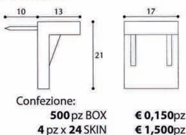
Art. 42063 Mensola pratica a due punti colori: bianco, marrone
