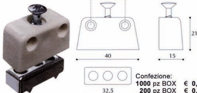
Art. 42039 Giunzione d'assemblaggio colori: bianco, marrone
