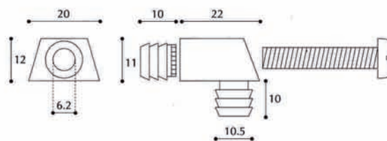
Art. 42096 Traplex colori: bianco, marrone
