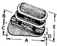
Art.PIO15 Piede ovale inclinato 15x30
