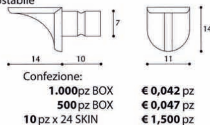
Art. 42019 Bussola per mensola spostabile colori: bianco, marrone
