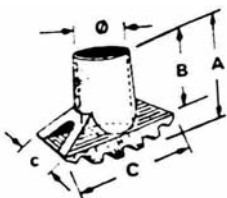
Art.PSAR Piede scala artiglio ø 32-35-38-40
