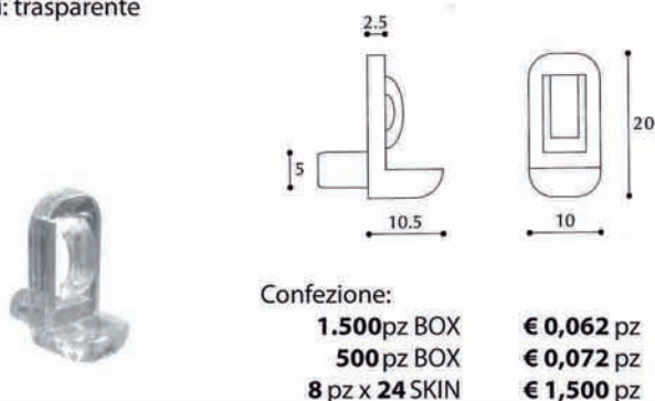
Art. 42196 Reggicristallo antiribaltamento colori: trasparente
