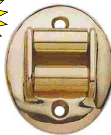
Art.82316 Guidacinghia lusso materiale: ottone mm. 62x52 Box 24 pz. Skin pz.1x24 O.L. € 6,50 € 7,50 O.BR. € 7,50 € 8,50 CR. € 7,50 € 8,50 CR/SAT € 8,80 € 9,80
