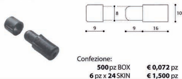
Art. 42122 Catenacciolo colori: bianco, marrone
