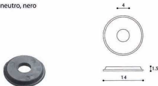
Art. 42046 Rondella colori: neutro, nero
