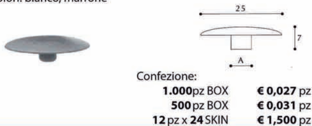
Art. 42007 Placca copri serrature colori: bianco, marrone
