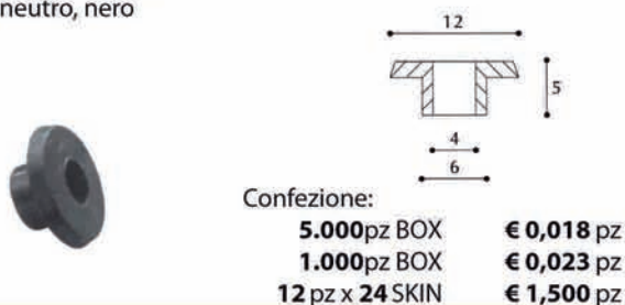
Art. 42045 Sottovite con bordo colori: neutro, nero
