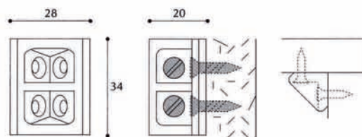
Art. 42040 Giunzione angolare colori: bianco, marrone
