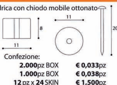
Art. 42030B Mensola cilindrica con chiodo mobile inserito ottonato colori: bianco, marrone
